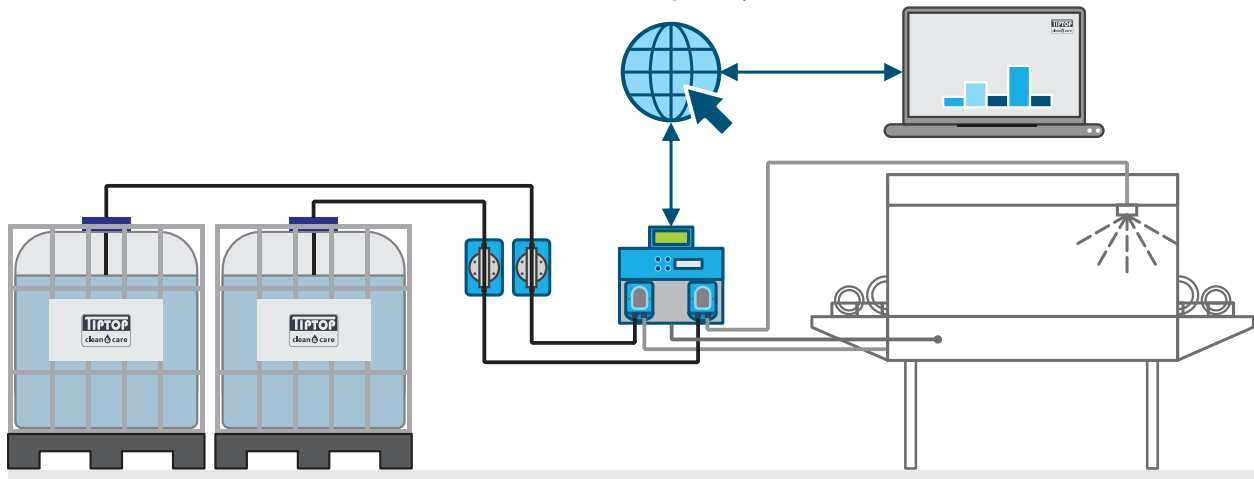
Große Geschirrspülersysteme
